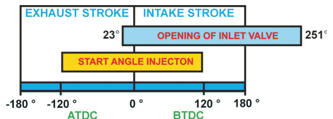
Rys. 3. Zakres zmian kąta początku wtrysku
